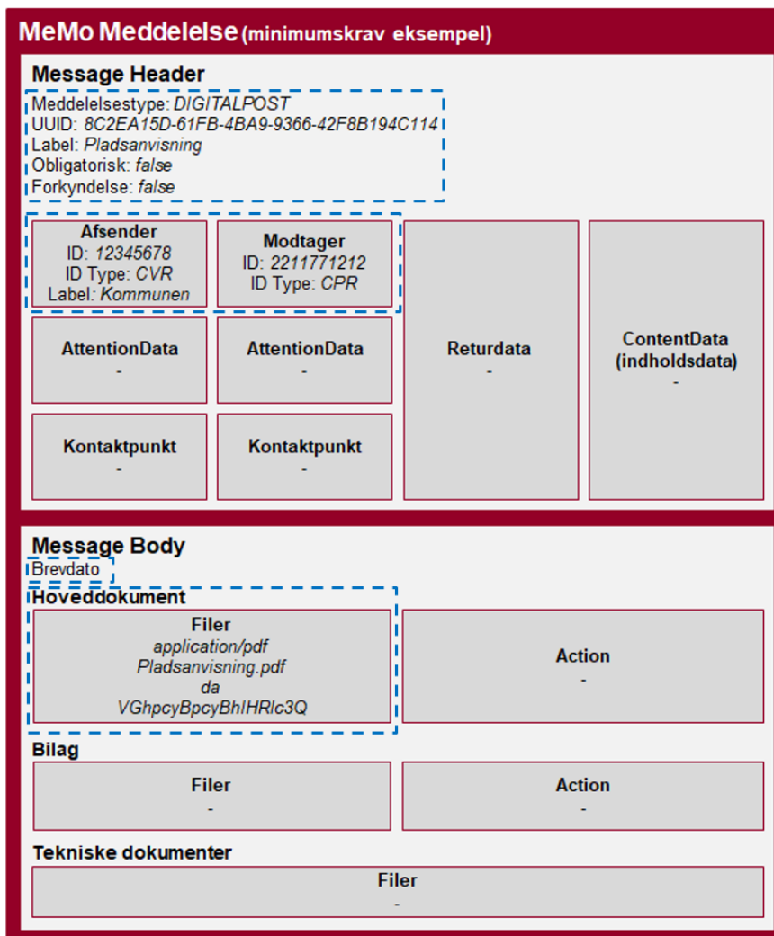
Figur 1. Illustration af strukturen for opmærkning med MeMo.
