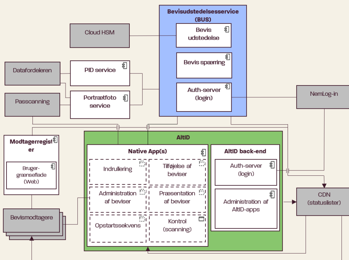
Figur 7: Højniveauarkitektur
